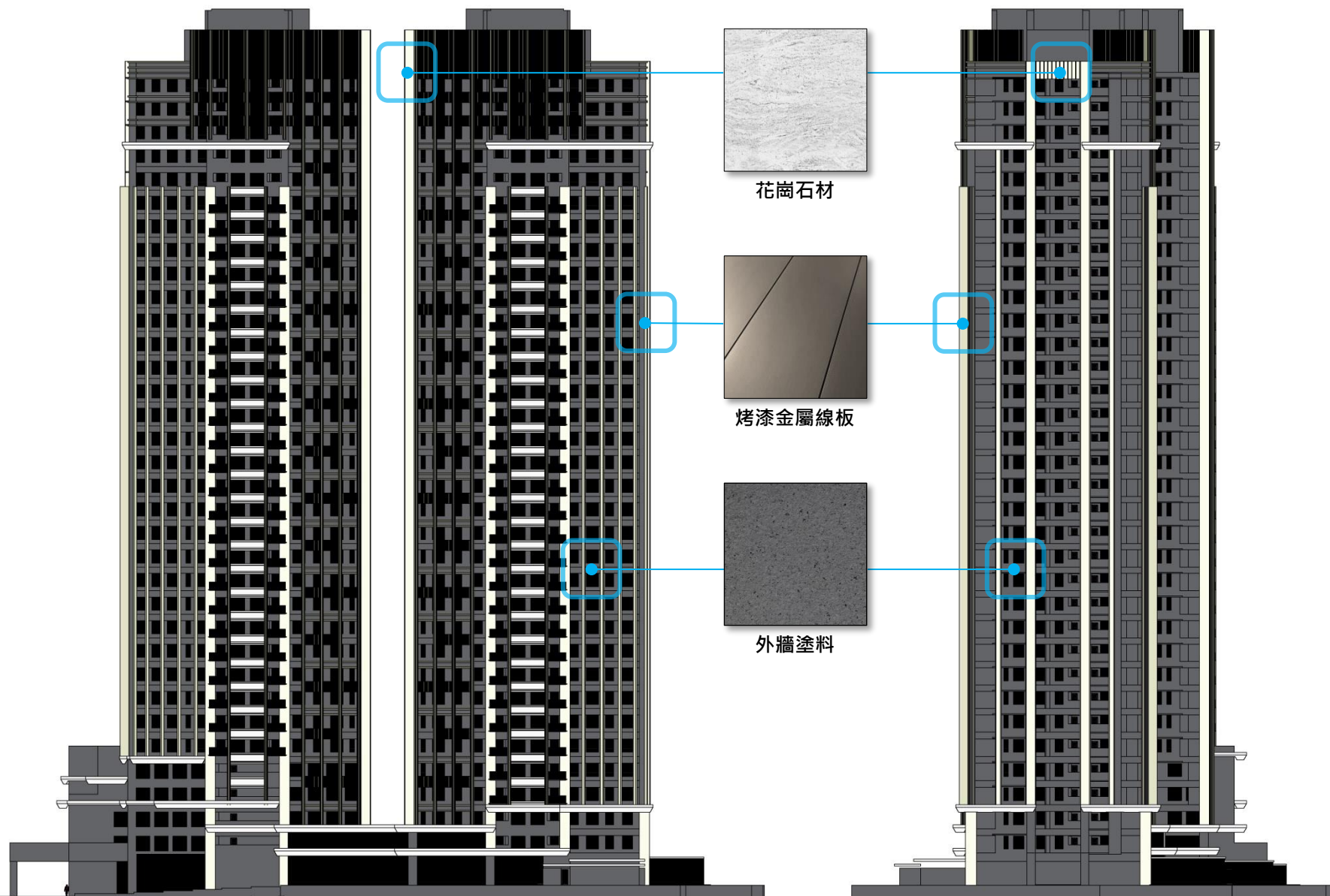
北向立面圖
