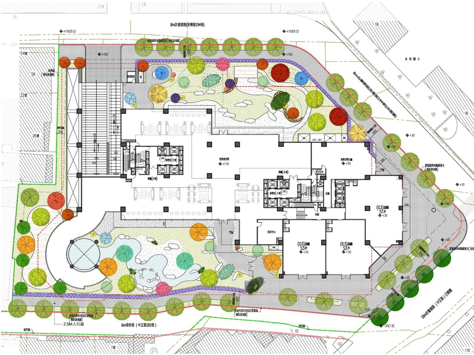
壹樓綠化平面圖
