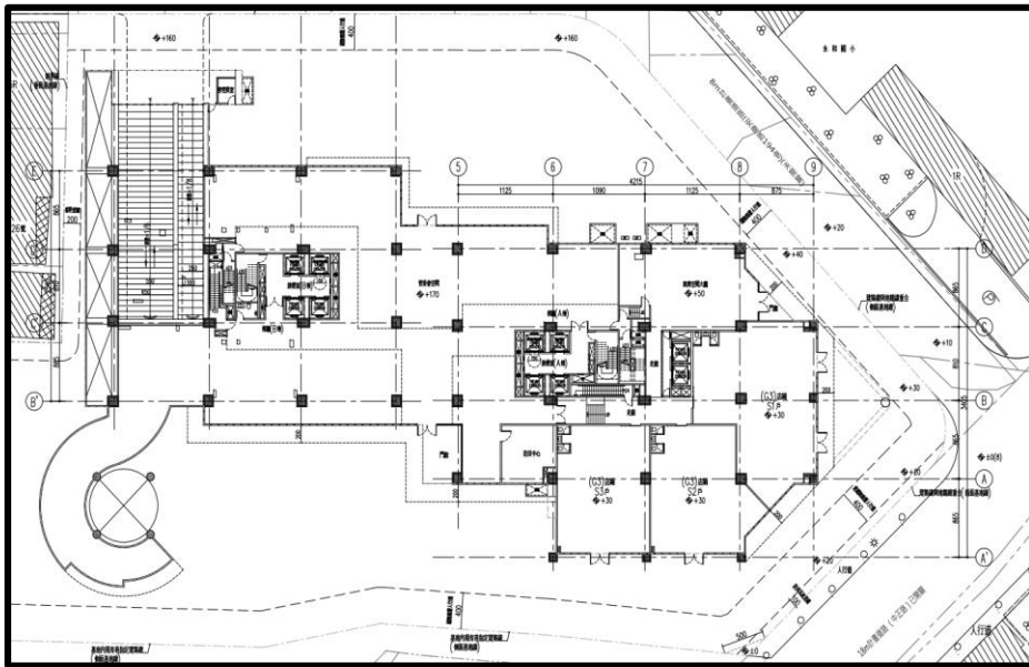
一樓平面圖
