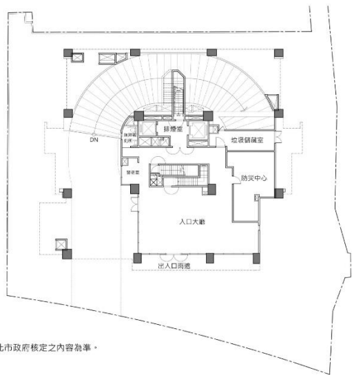
擬訂新北市中和區公園段 443 地號等 12 筆土地都市更新權利變換計畫案 建物及停車位位置編號圖
