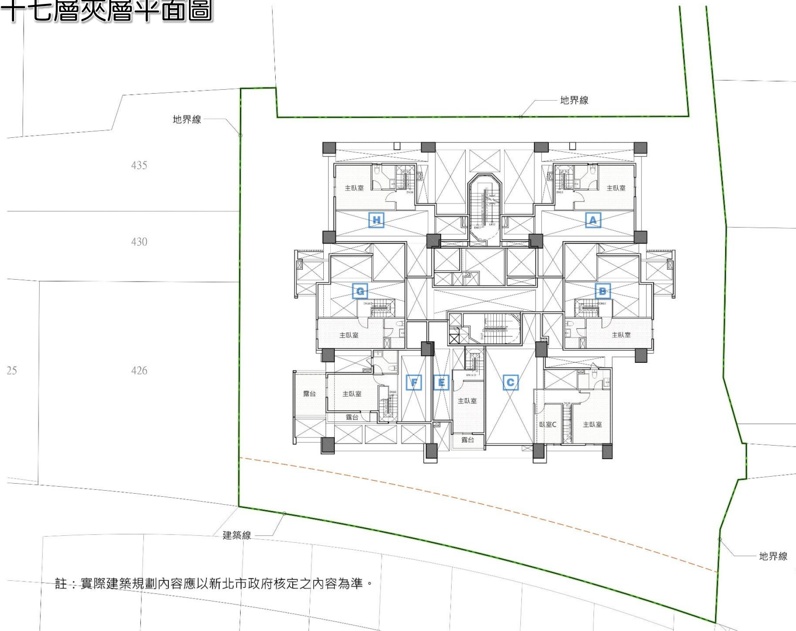
十七層夾層平面圖
