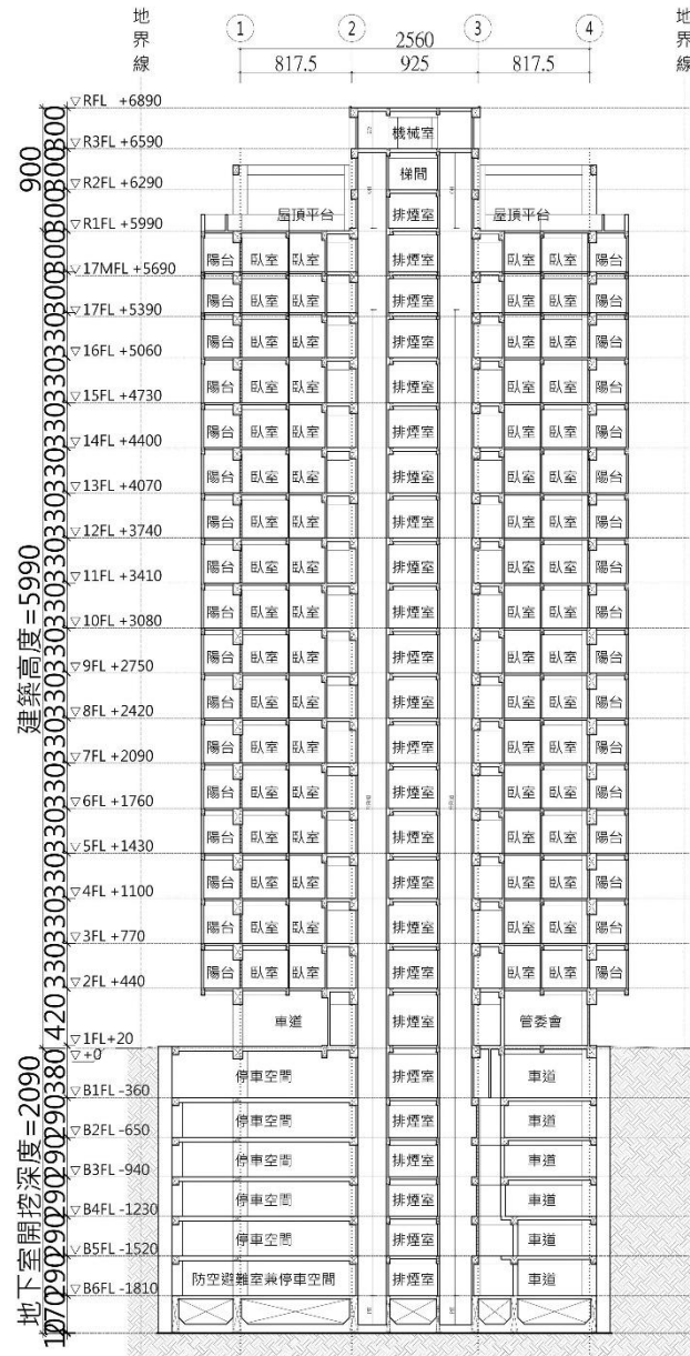
剖面圖(一)
