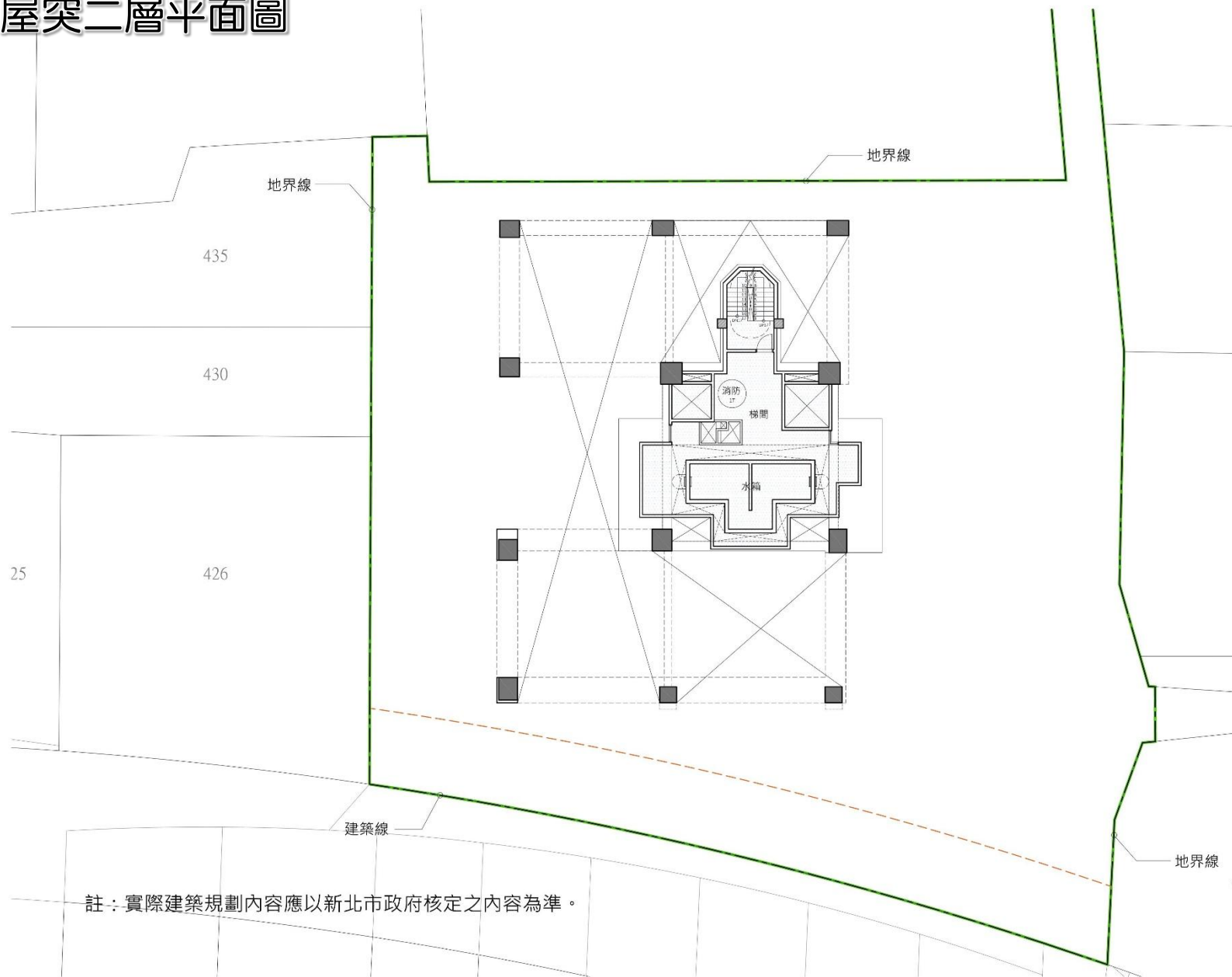
屋突二層平面圖
